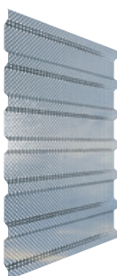
Kalzip TR 30/167 P
